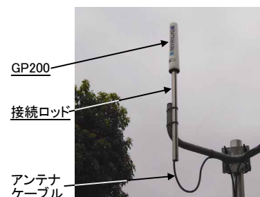
GP200 設置例
