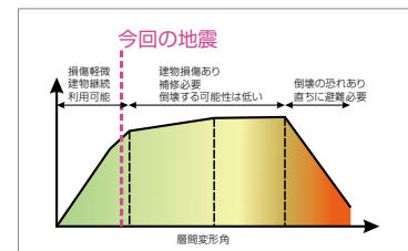
建物層間変形角評価結果
